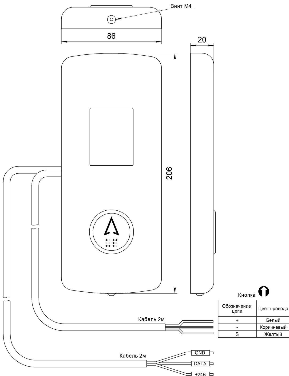
Рис.1 Внешний вид, габаритные и установочные размеры Вызывного поста ВП-1101-1074-07
